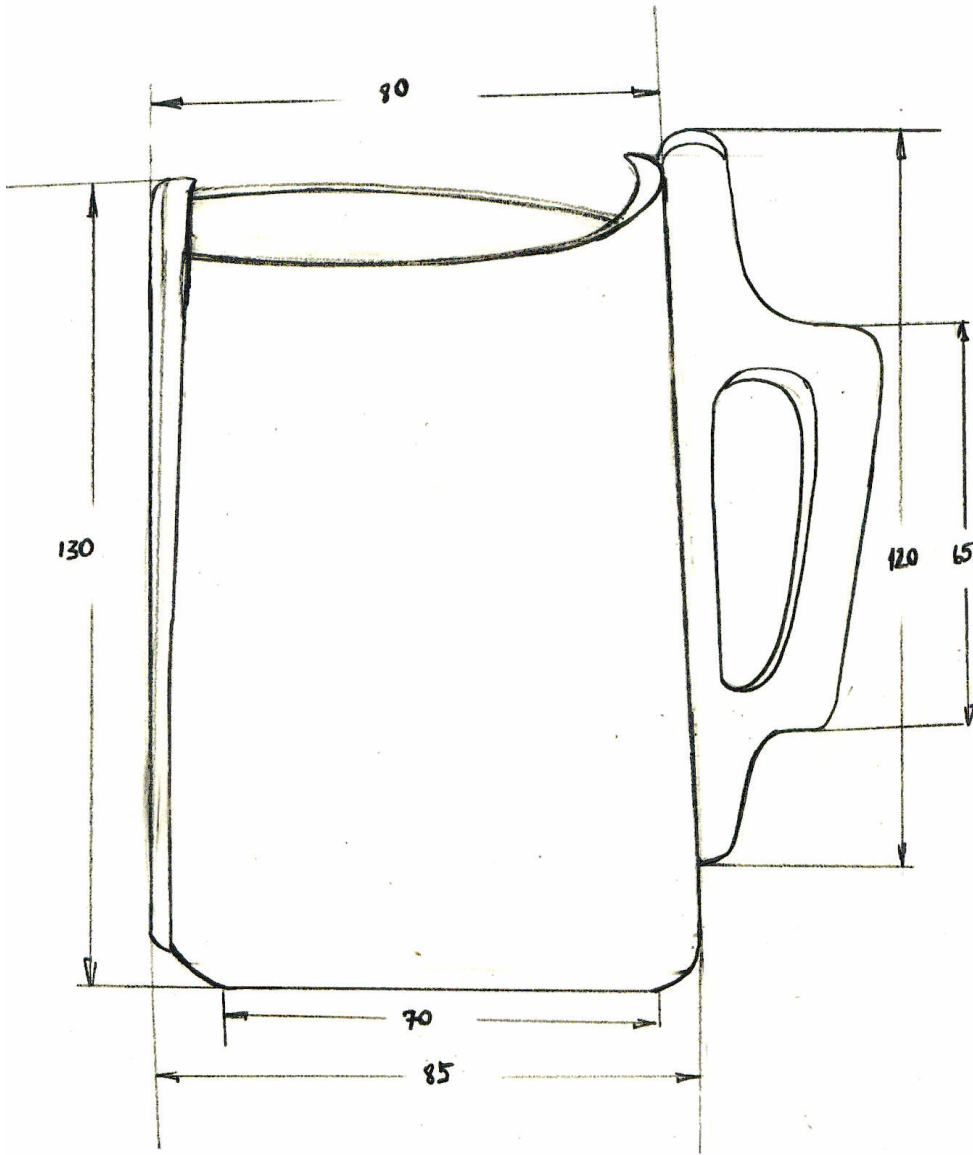
Şekil 1.27: Gerçek ölçüsünde çizilmiş kupa tasarımı
