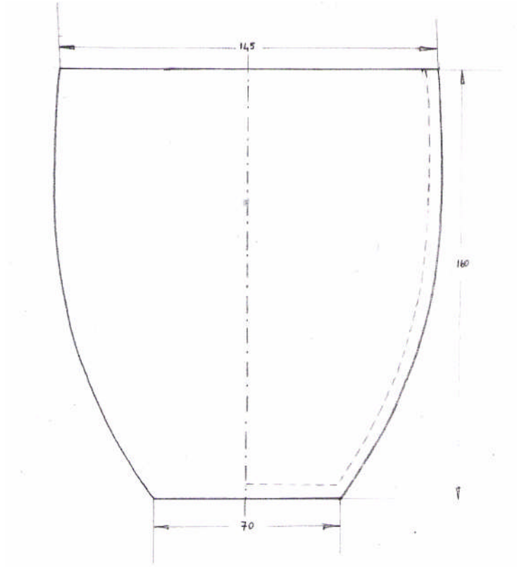
Şekil 1.25: ½ ölçeğinde çizilmiş saksı tasarımı
