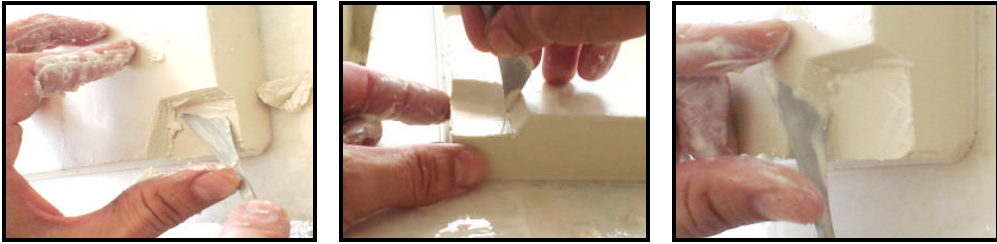
Resim.5.6: Alçı plaka köşesinde köşeli pim açma aşamaları
