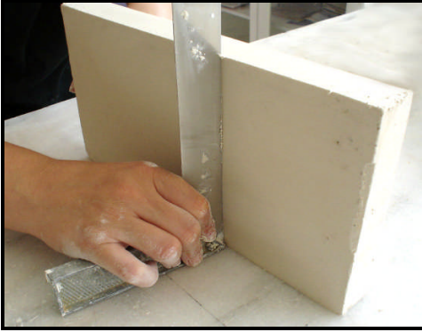
Resim4.9: Alçı plaka yüzeyi ölçü kontrolü
