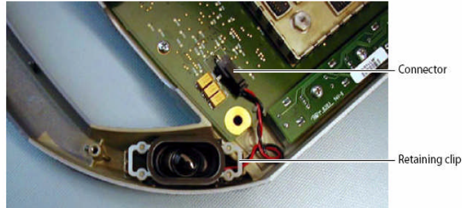
Şekil 1.3: Hoparlörün değiştirilmesi
