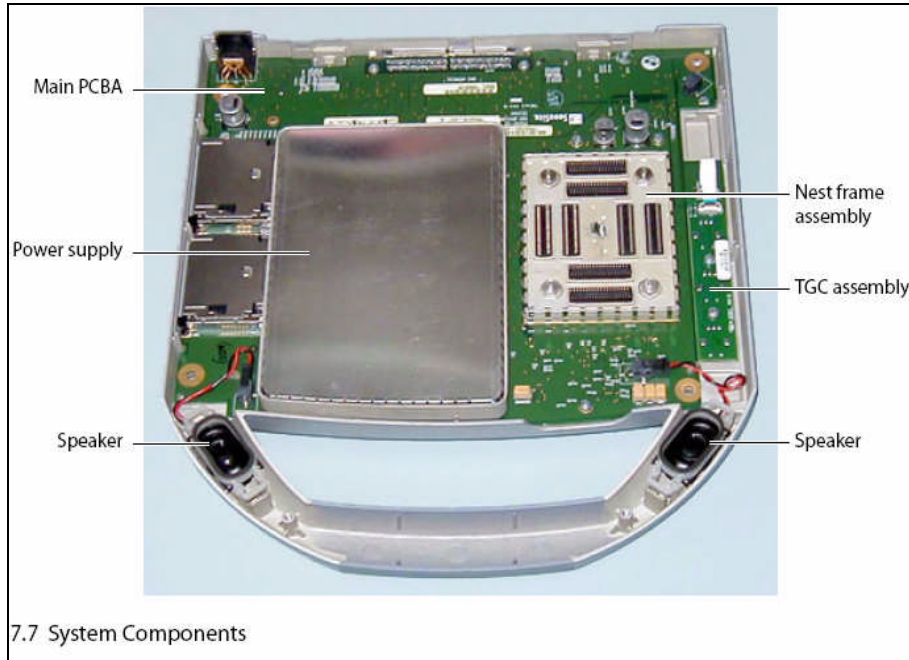
Şekil 1.2: Bir ultrason sisteminin ana sistem bileşenler
