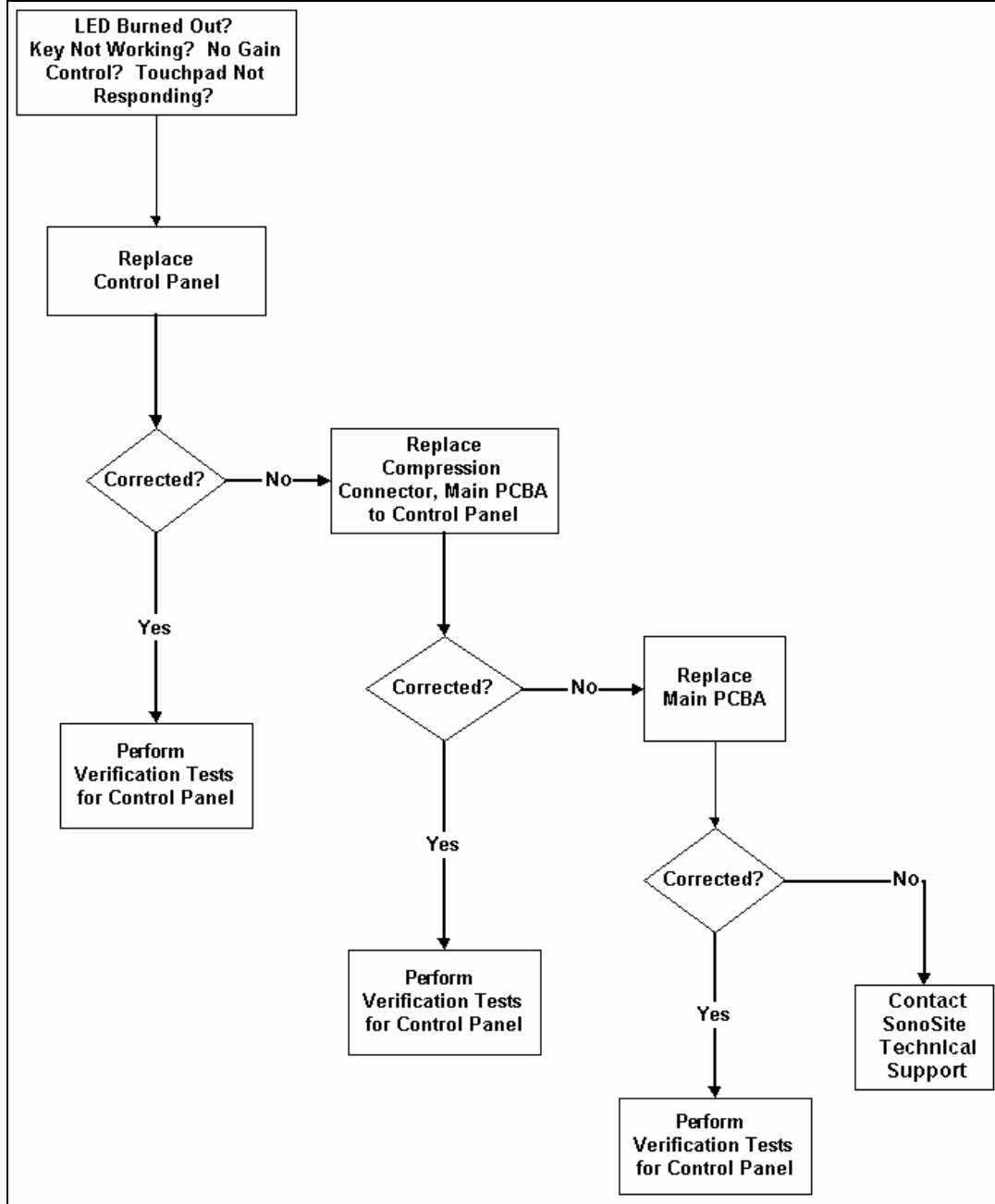
Bir ultrason sisteminde kontrol paneli arızası için akış diagramı
