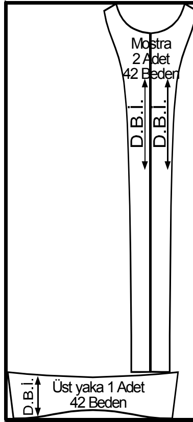
Şekil 2: Tela eni 90cm Tela kalıplarını açık enli olarak telaya yerleştirme
