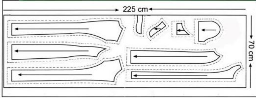
Şekil 1.1: Kumaş yerleşim planı
