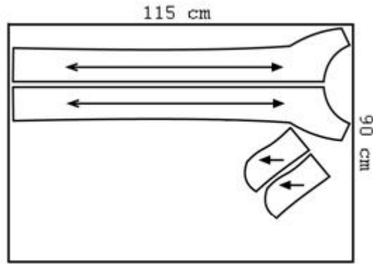
Şekil 1.2: Tela yerleşim planı
