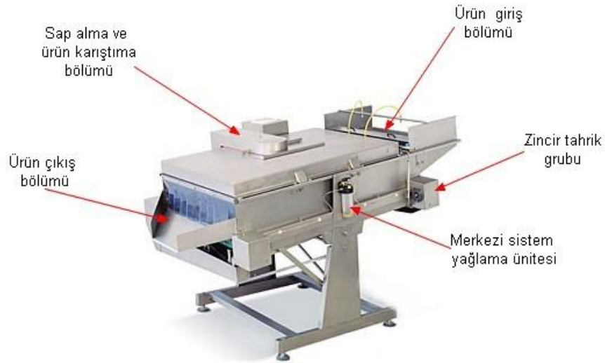
Resim 1.5: Sap alma makinesinin kısımları
