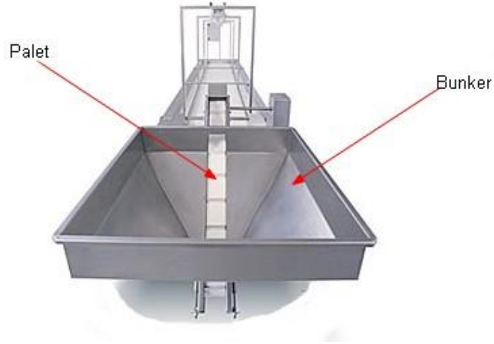
Resim 2.3: Seçme bandının besleme ünitesi (bunkeri)
