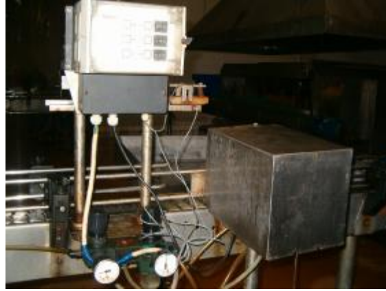
Resim 3.21: Vakum dedektörü
