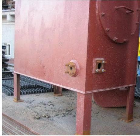
Resim 1.5: Ayak (support) uygulaması
