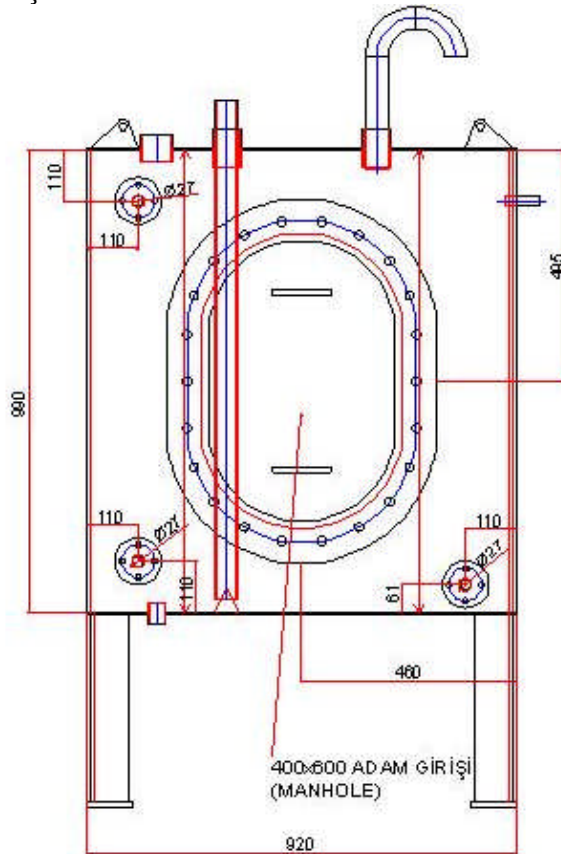
Şekil 1.5: Tank ön görünüşü (front view)
