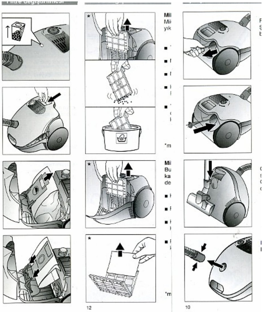
Resim 1.1: Elektrik sprgesinin temizlik ve bakımı
