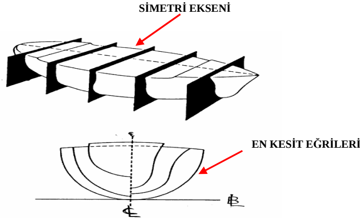
Şekil 1.1: En kesit alanları eğrisi
