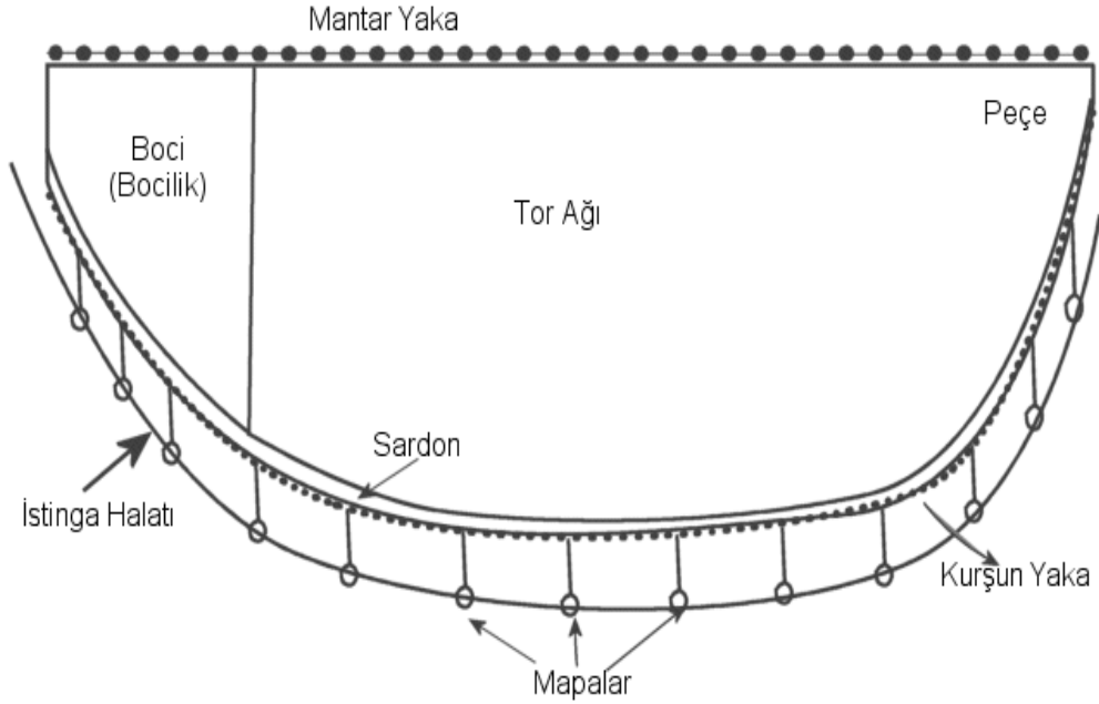
Şekil 4: Gırgır ağı
