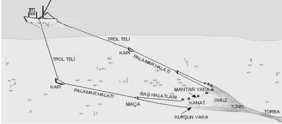
Şekil 2: Trol ağının genel yapısı
