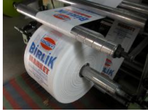
Resim 1.6: Bir tarafı sabit sargı ünitesi
