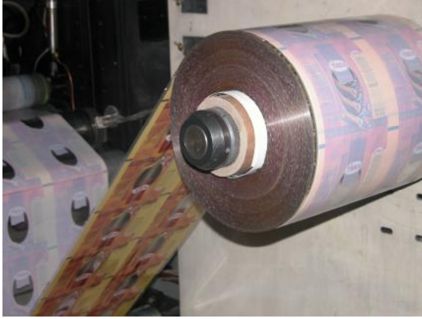
Resim 1.2: Sargı işlemi
