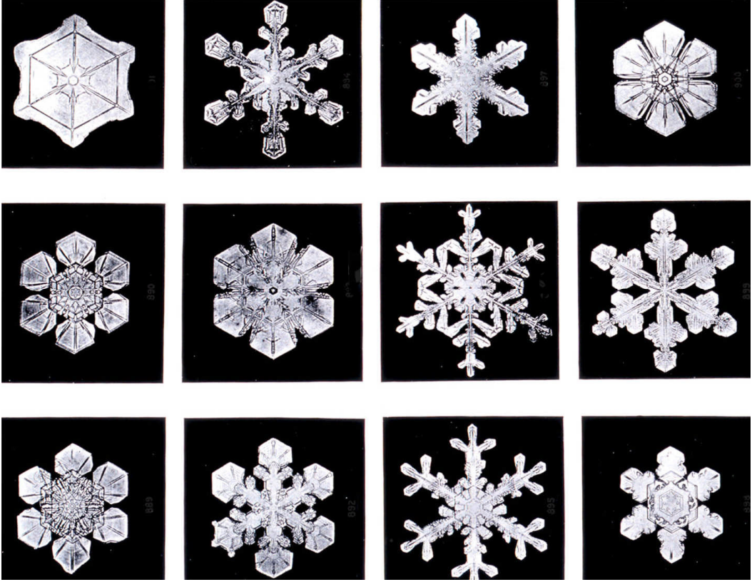
Resim 1.10: Kar kristalleri
