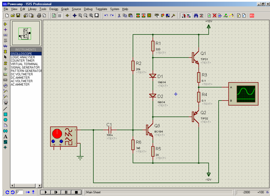
Şekil 5.8. Osilaskop ve sinyal jeneratörünün şemaya eklenmesi
