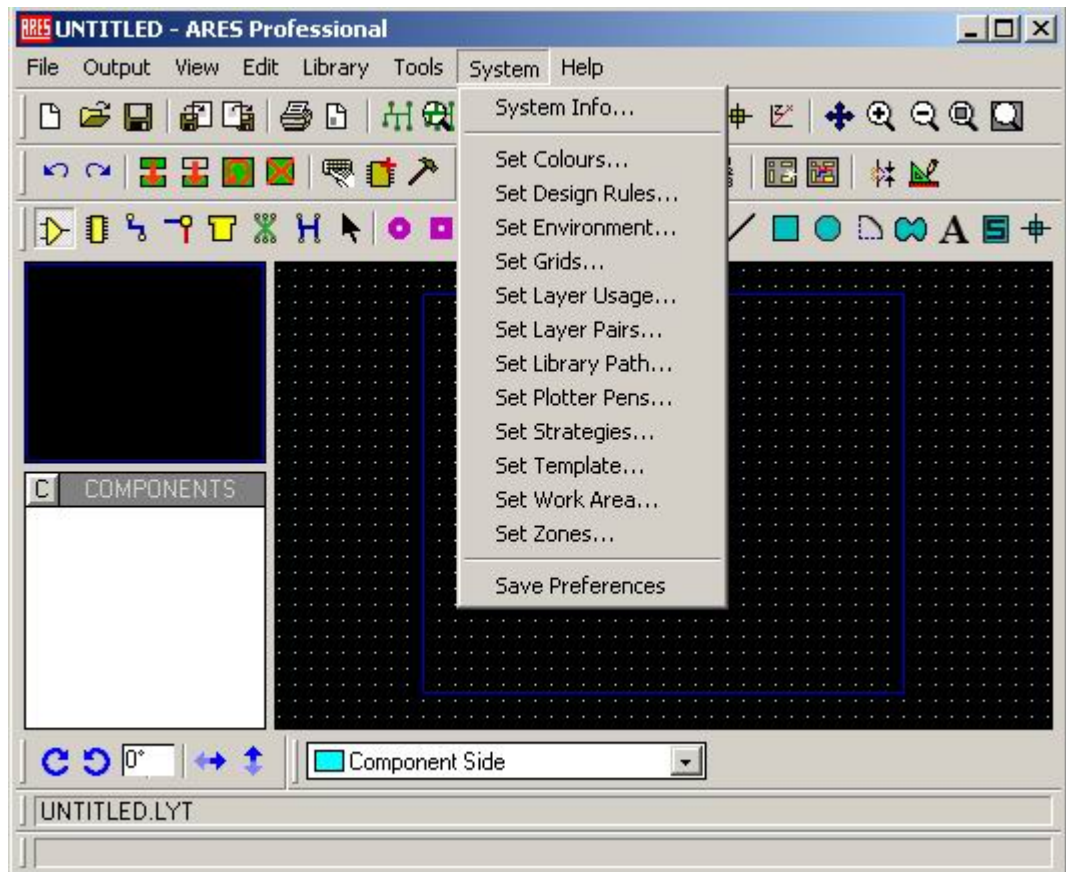
Şekil 4.47. System menüsü
