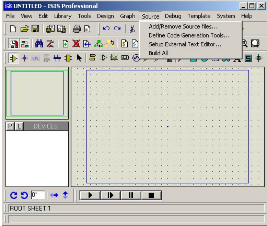
Şekil 3.35. Source menüsü
