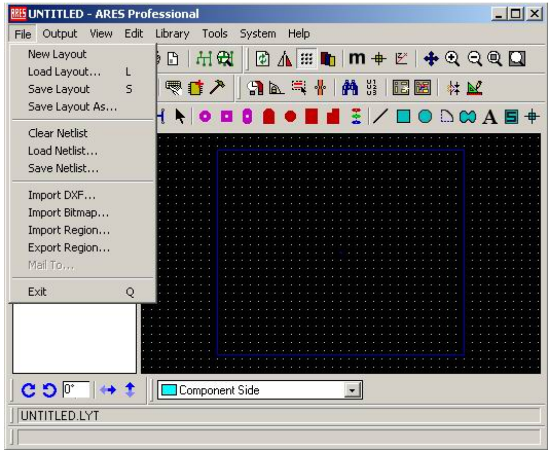
Şekil 4.10. File menüsü
