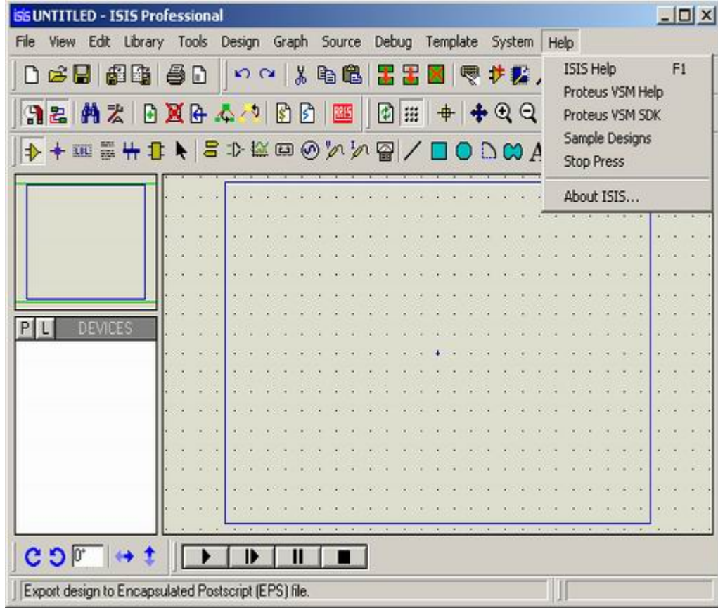
Şekil 3.55. Help menüsü
