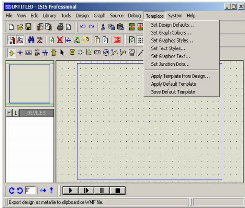
Şekil 3.40. Template menüsü
