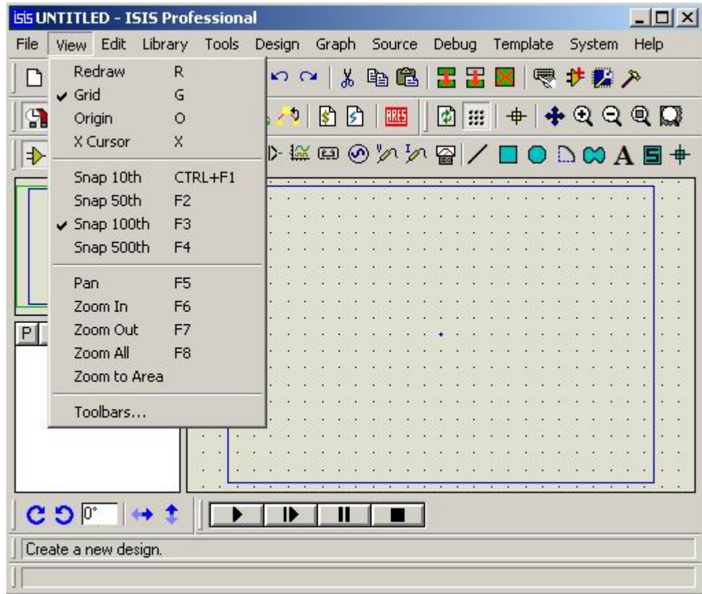
Şekil 3.12. View menüsü
