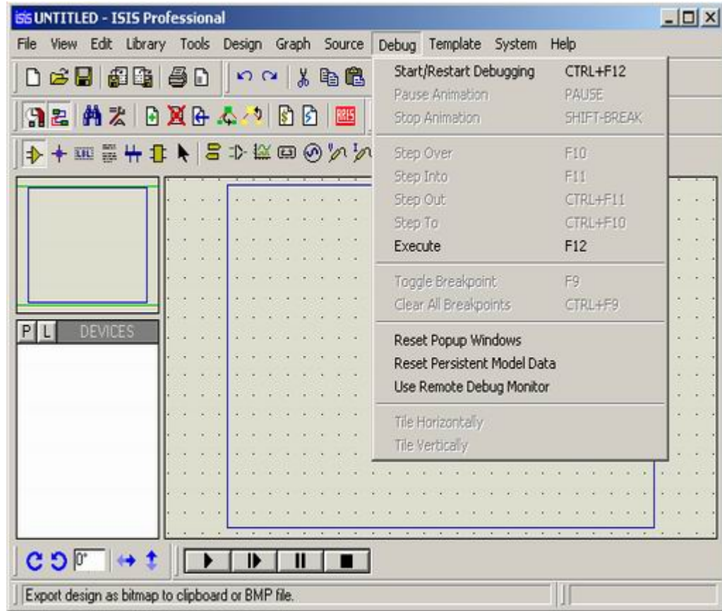
Şekil 3.39. Debug menüsü
