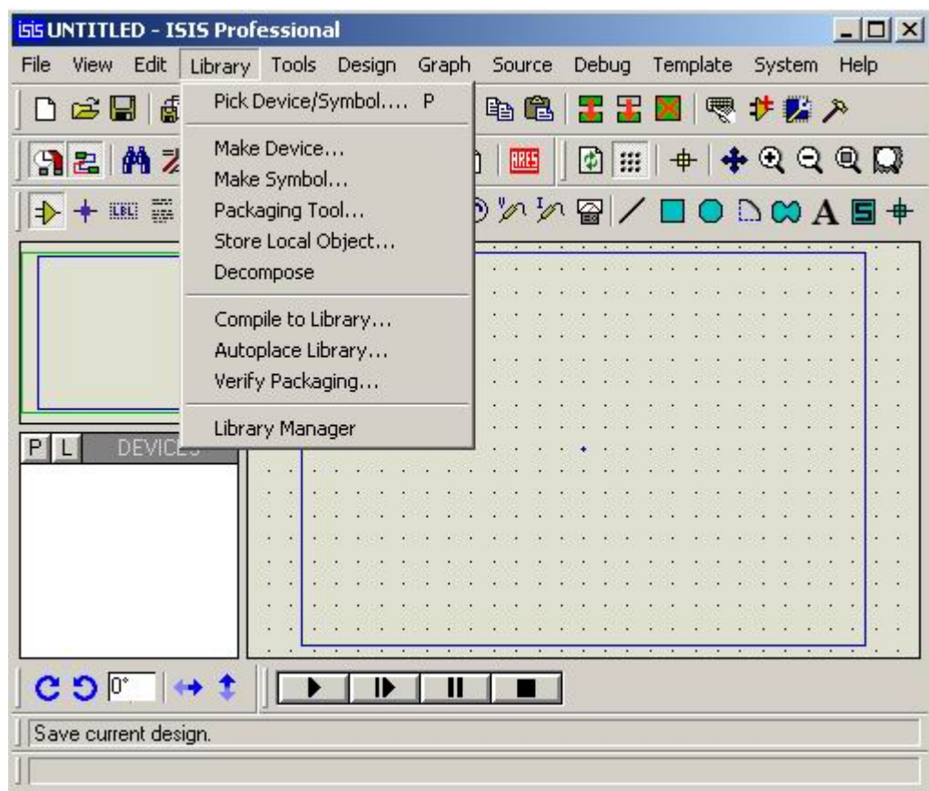
Şekil 3.15. Library menüsü
