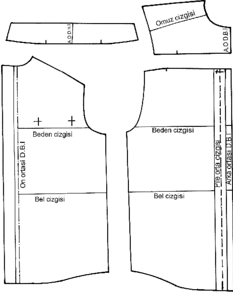
Şekil 1.3 Erkek gömleği yaka, roba, ön ve arka beden açılımları
