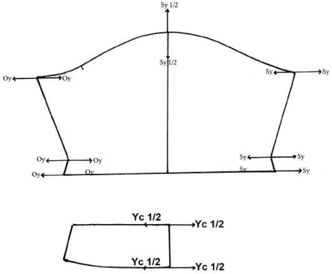
Şekil 2.2: Erkek gömleği kol ve yaka sıçrama noktaları ve yönleri
