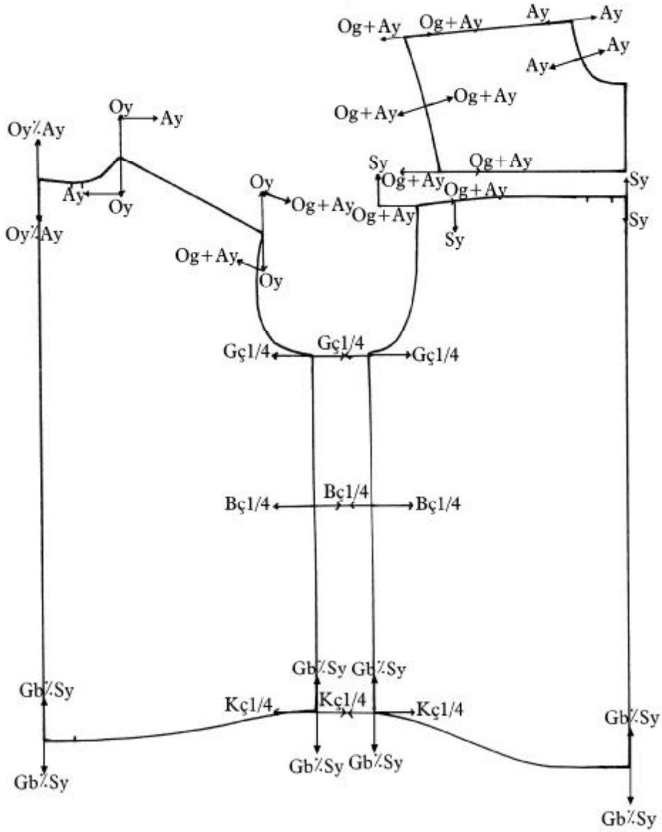
Şekil 2.1: Erkek gömleği roba, ön ve arka beden sıçrama noktaları ve yönleri
