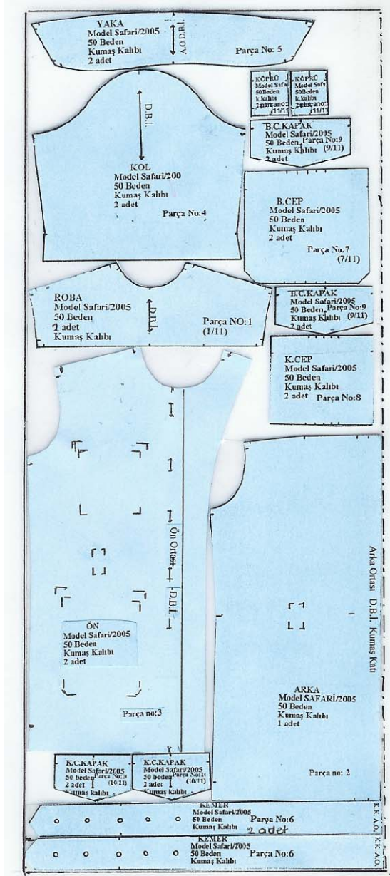
Şekil 2.1: Çift en kumaşa kalıbı (katlı şekilde) yerleştirme (yarım pastal)
