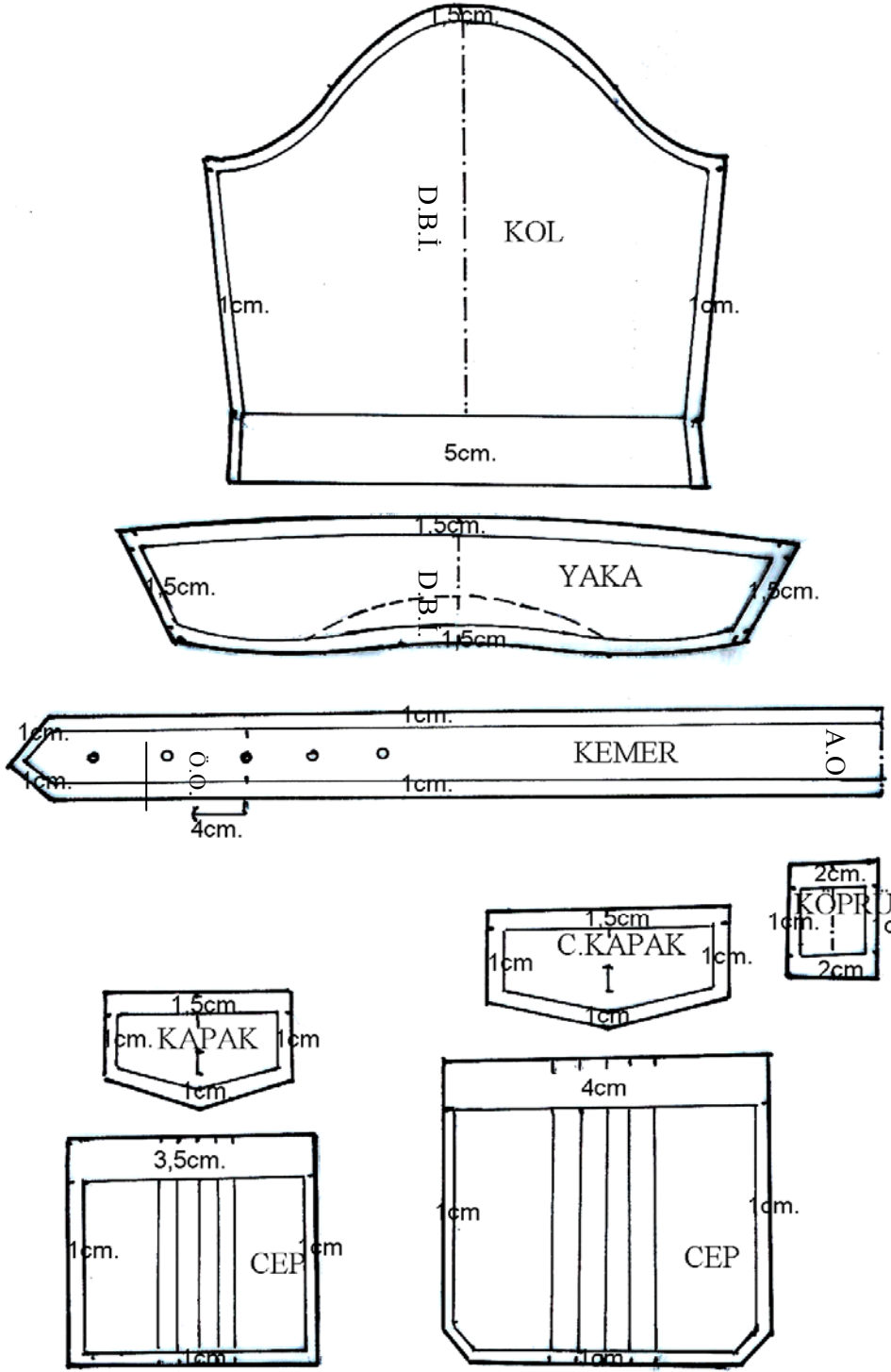
Şekil 1.6: Safari gömlek şablonlama (kol - yaka - kemer - cepler)
