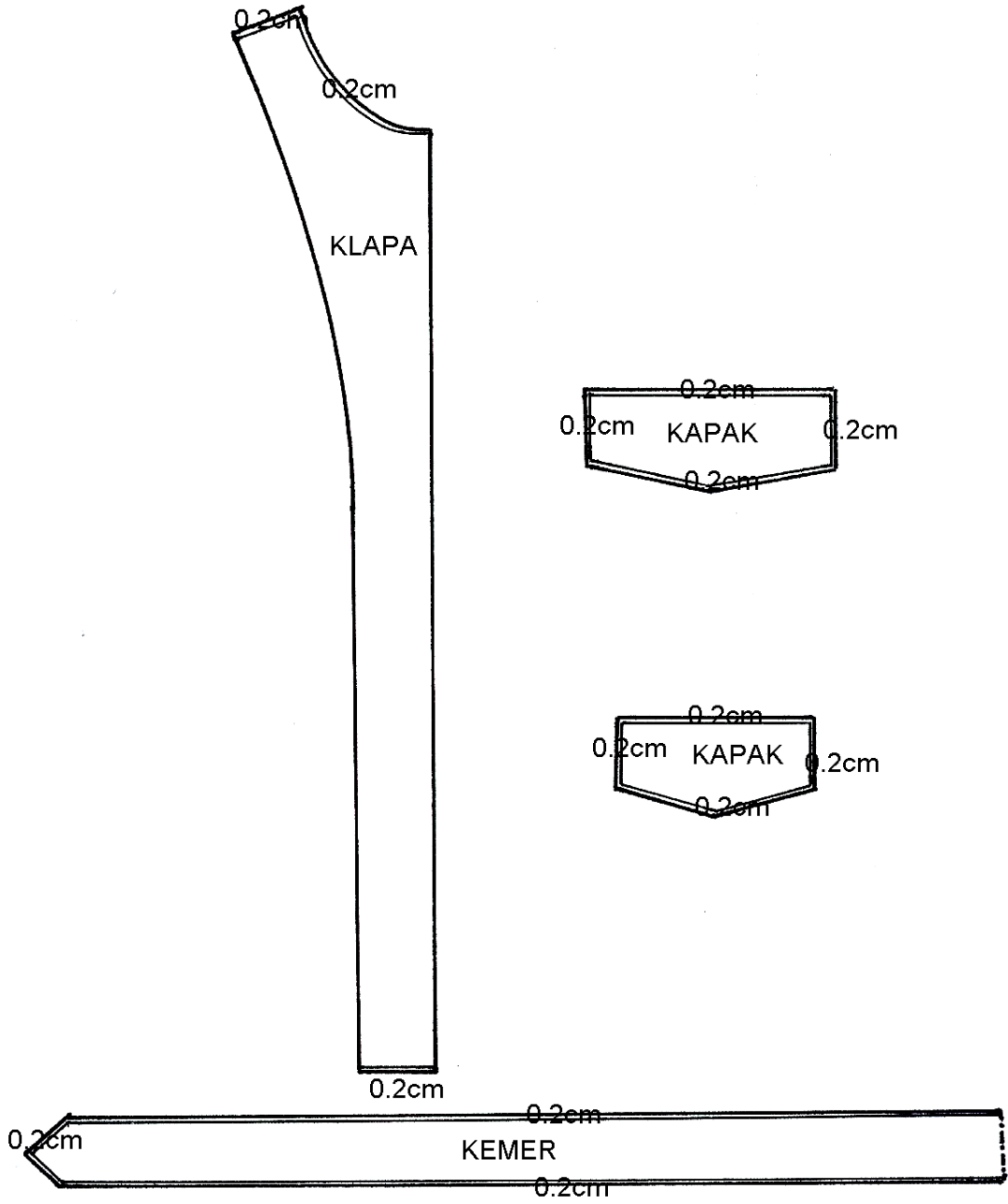
Şekil 1.7: Safari gömlek tela şablonu hazırlama
