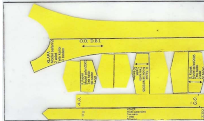
Şekil 2.3: Tela metraji hesaplama
