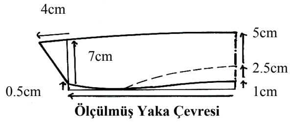
Şekil 1.2: Safari gömlek model uygulama (kol – yaka)
