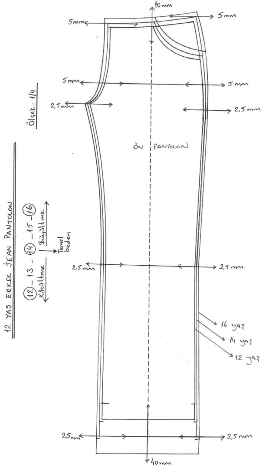
Şekil 2.4: Ön pantolon seri çizimi
