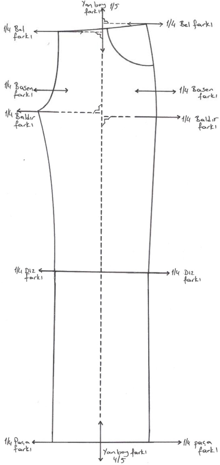
Şekil 2.1: Ön pantolon sıçrama noktaları ve yönleri
