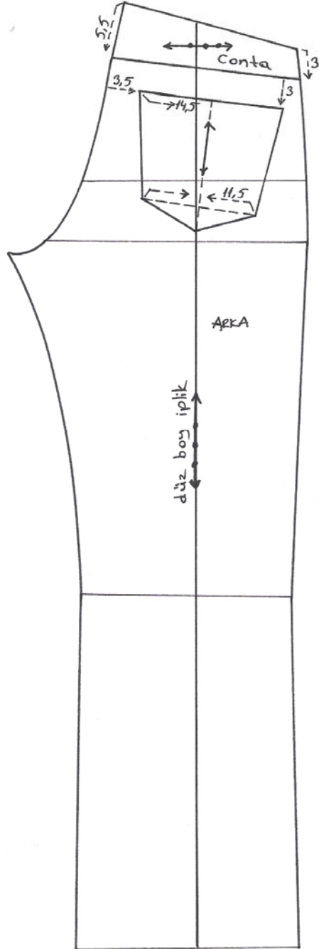
Şekil 1.8: Arka pantolon model uygulama
