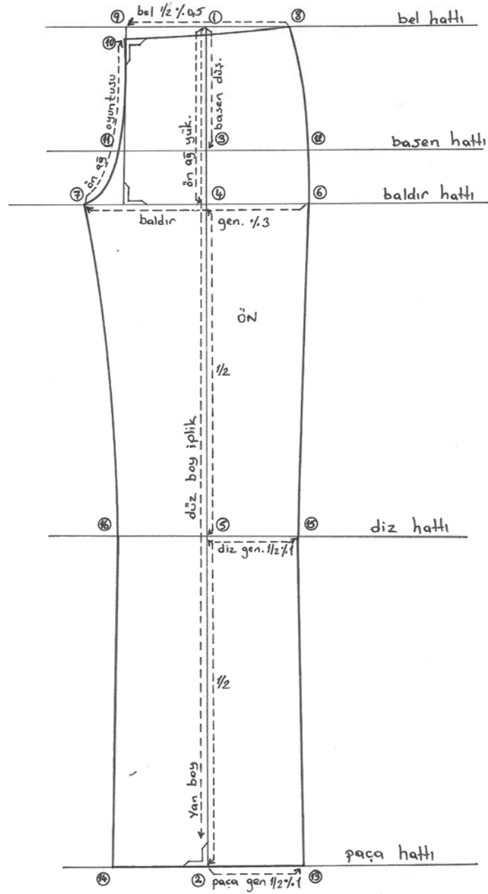
Şekil 1.5: Ön pantolon kalıbı çizimi
