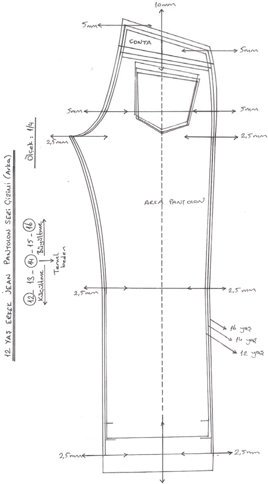
Şekil 2.6: Arka pantolon seri çizimi
