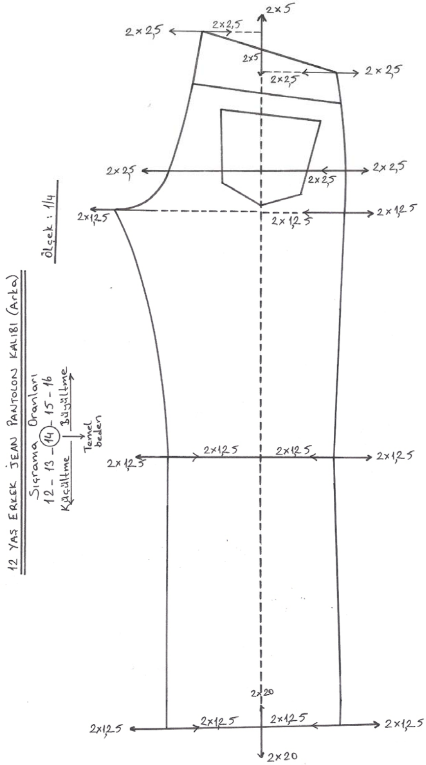
Şekil 2.5: Arka pantolon sıçrama oranları
