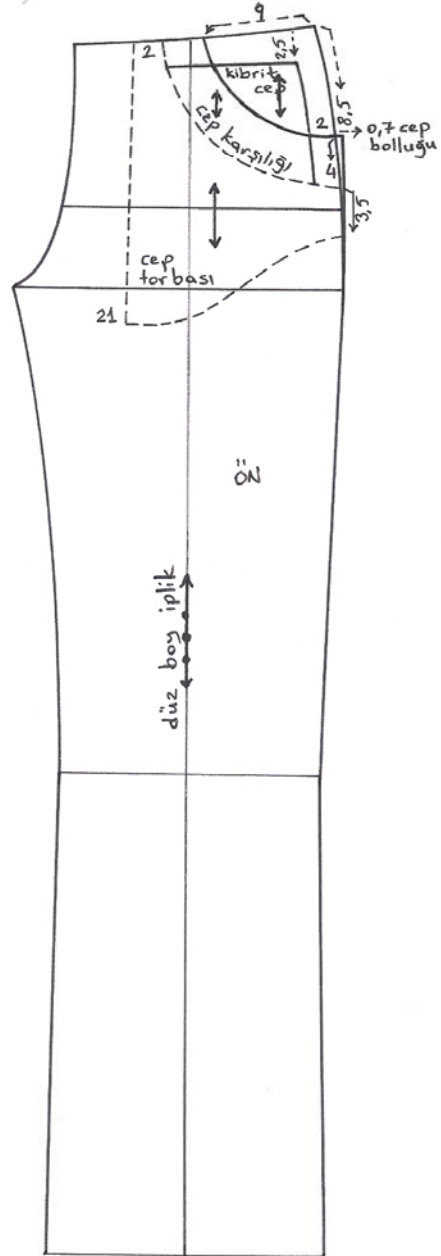
Şekil 1.7: Ön pantolon model uygulama
