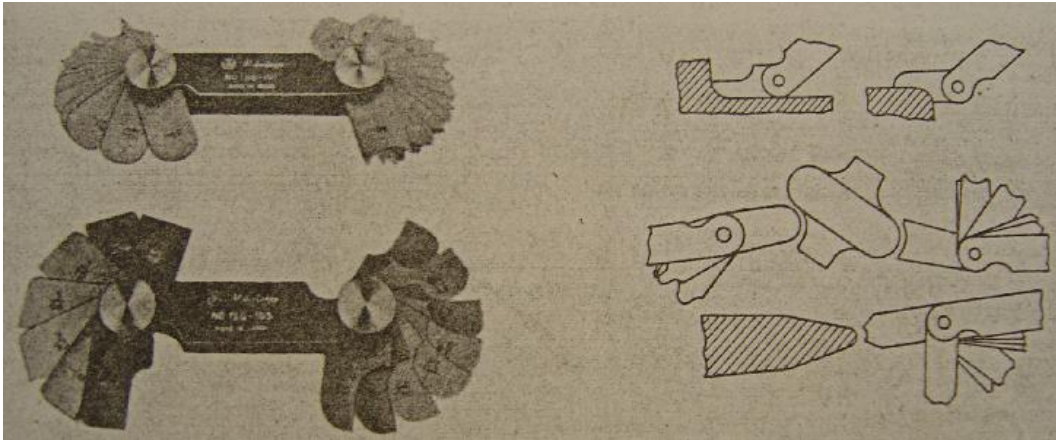
Resim 3.1: Profil mastarları
