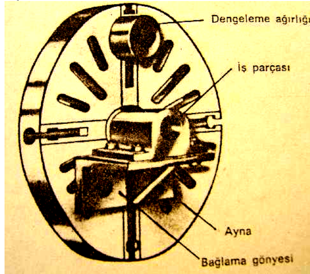
Şekil 2.1: Düz aynada gönye ile iş bağlama
