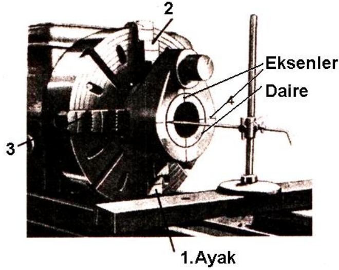
Resim 1.1: Mengenele aynada merkezleme
