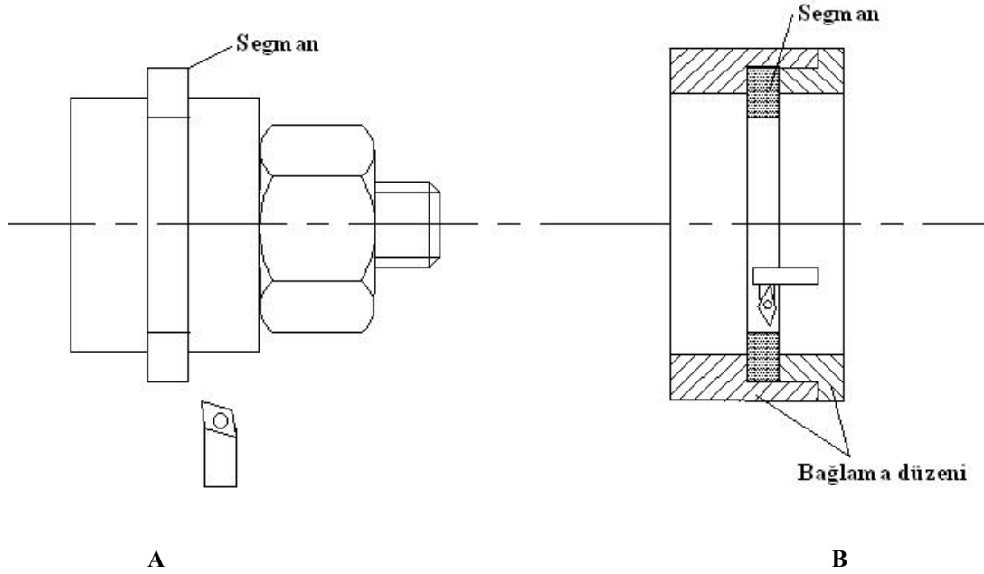
Şekil 3.5: Madeni segmanların A-Dış çapını tornalama B-İç çapını tornalama
